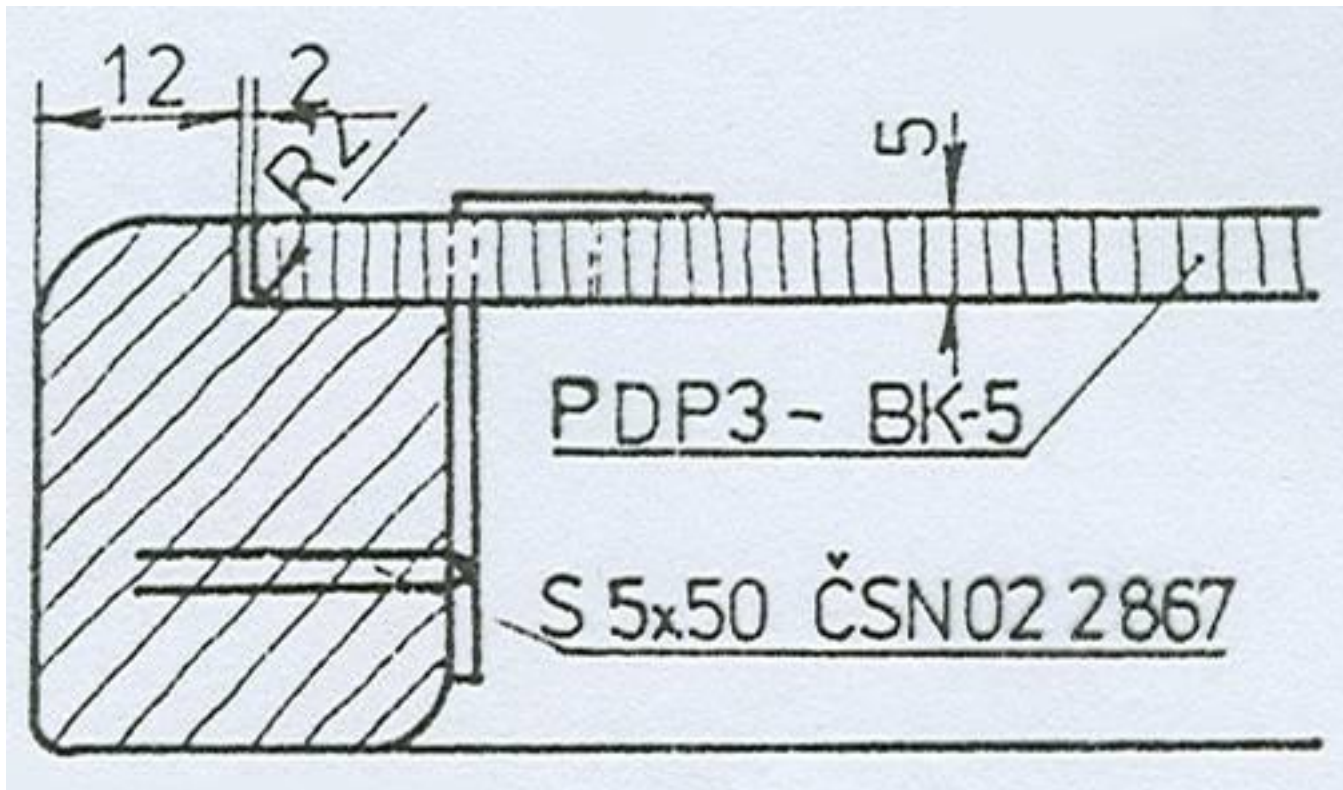
Upevnenie k lubom/rámu - uholník
